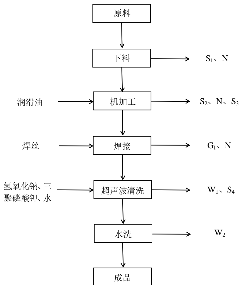
图 5-1 五金制品生产工艺及产污环节图
