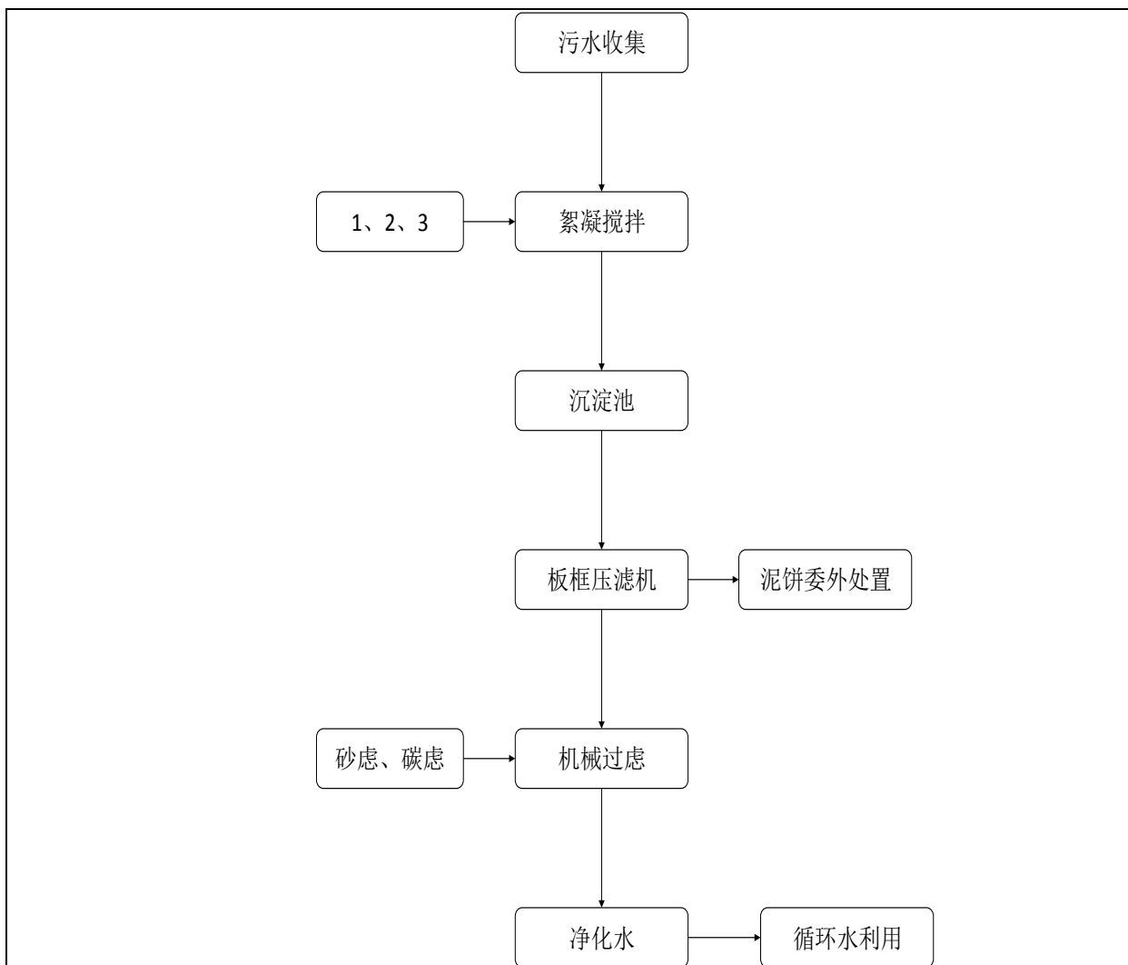
图 7-1 清洗废水处理工艺流程图
