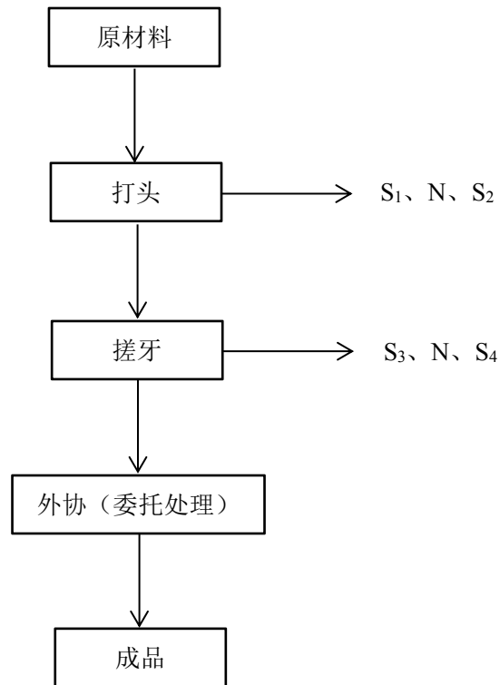
图 5-1 螺丝生产工艺及产污环节图
