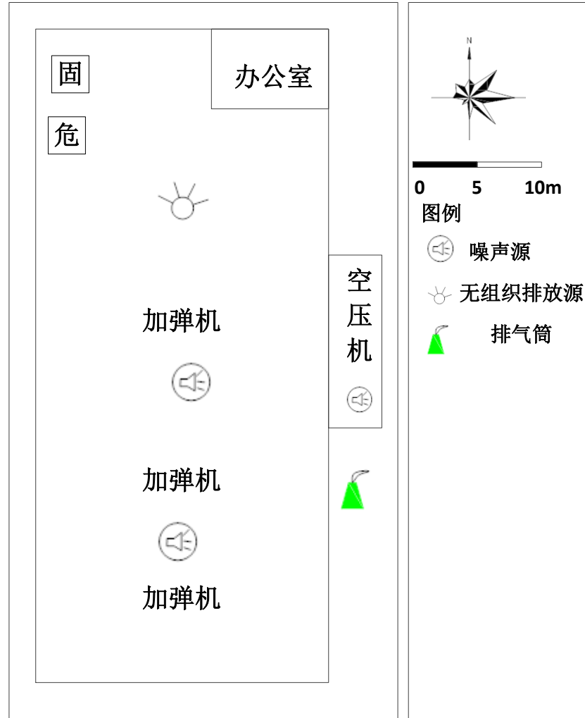
附图 3 厂区平面布置图
