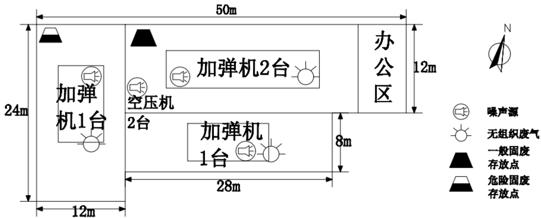
附图3 项目生产车间平面布置图
