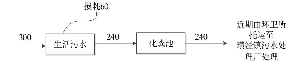
图 5-2 本次项目水平衡图 (t/a)
