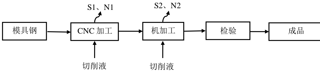
图 5-1 电镀设备工艺流程及产污环节图
