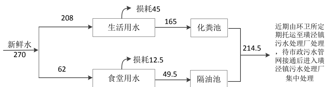
图 1-2 现有项目水平衡图 (t/a)
