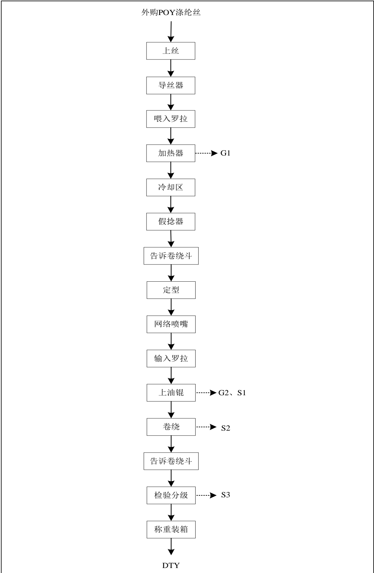
图 5-1 涤纶 DTY 加弹丝生产工艺流程及产污节点图
