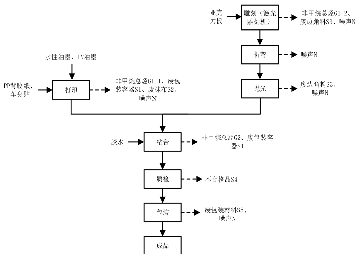
图 5-2 展示道具生产工艺流程图
