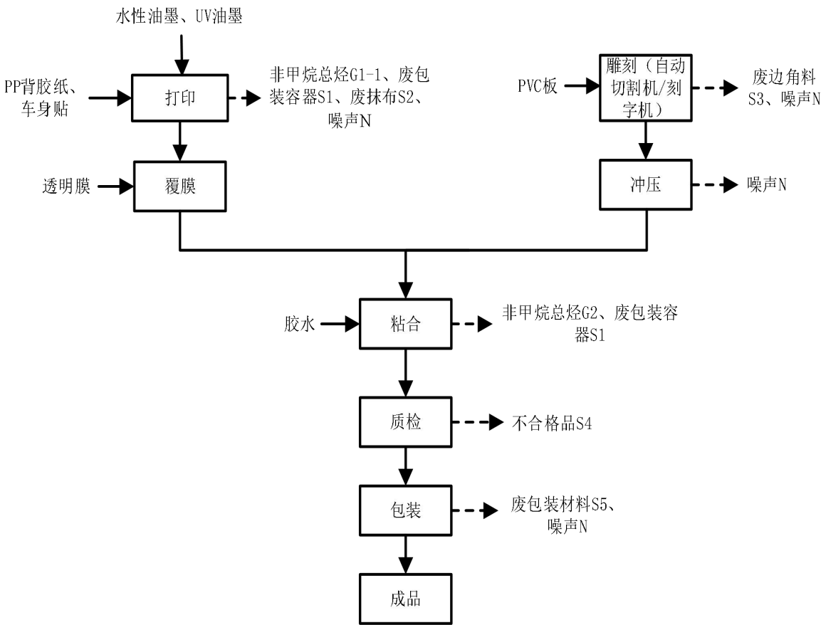
图 5-1 广告板、标识牌生产工艺流程图
