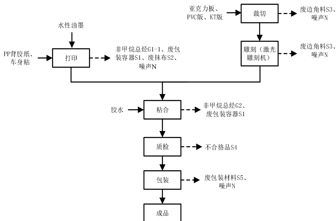
图 5-3 展示架生产工艺流程图
