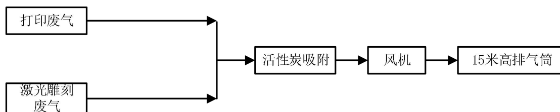
图 7-1 废气处理工艺流程图
