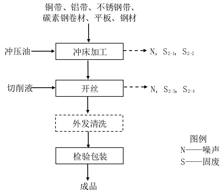
图 2 冲压、钣金件生产工艺流程图
