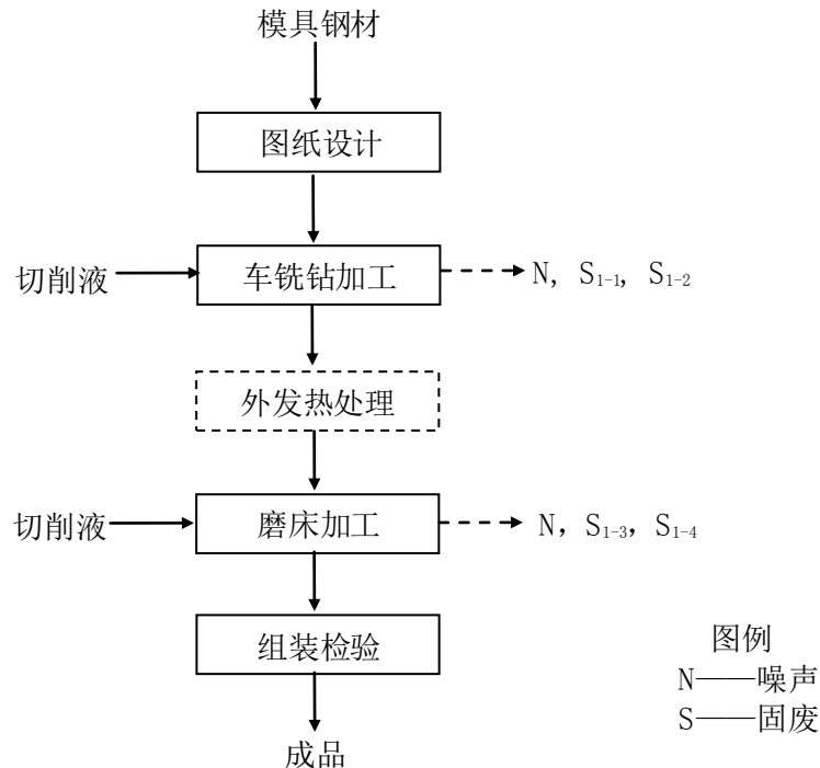
图 1 模具生产工艺流程图
