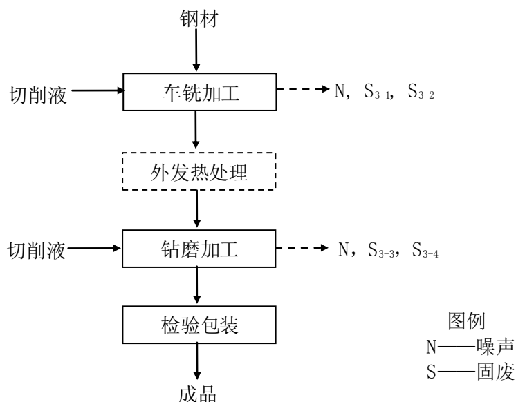
图 3 机械零部件生产工艺流程图
