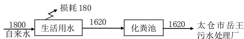
图 4 建设项目用排水平衡图（单位 t/a）
