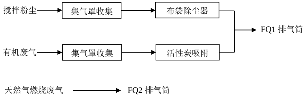
图 7-1 有组织废气处理整体流程示意图
