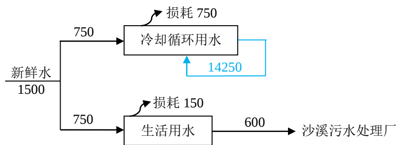
图 5-2 新建项目水平衡图 (t/a)
