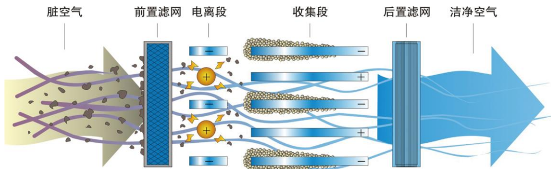
图 7-2 静电式油烟净化器流程示意图
