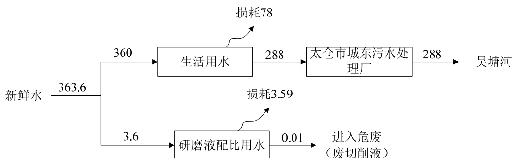
图 5-2 本项目水平衡图 (m³/a)
