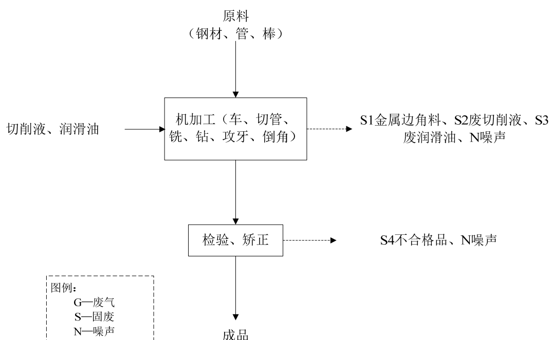
图 5-1 生产工艺流程图
