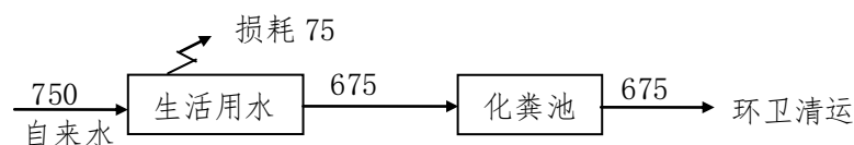
图 2 建设项目全厂用排水平衡图 (单位 t/a)
