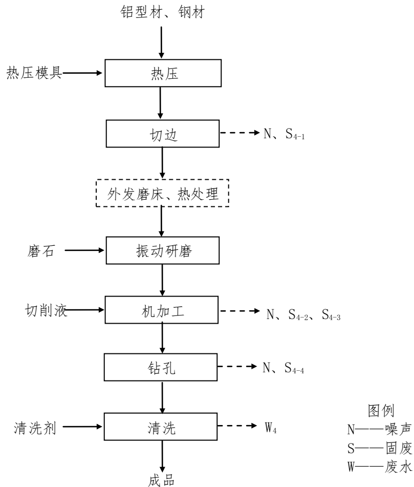
图 4 通用零部件（热压系列）生产工艺流程图
