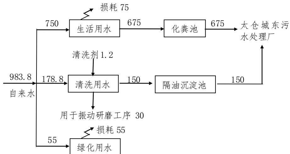
图 5 建设项目全厂用排水平衡图 (单位 t/a)
