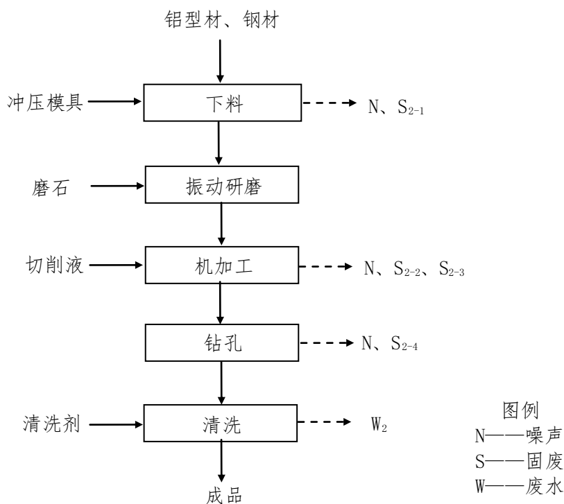
图 2 通用零部件（冲压系列）生产工艺流程图
