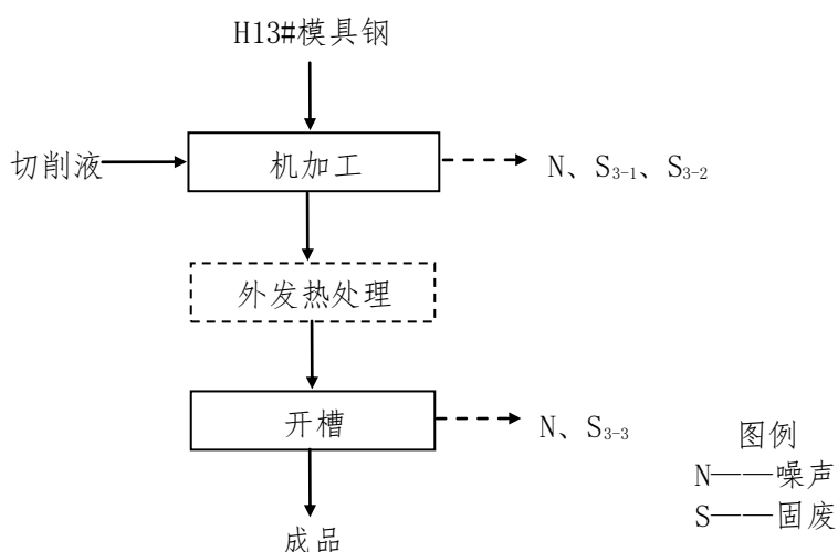
图 3 热压模具生产工艺流程图
