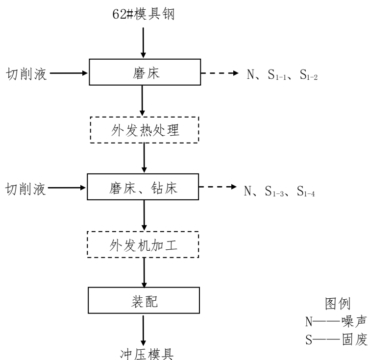
图 1 冲压模具生产工艺流程图
