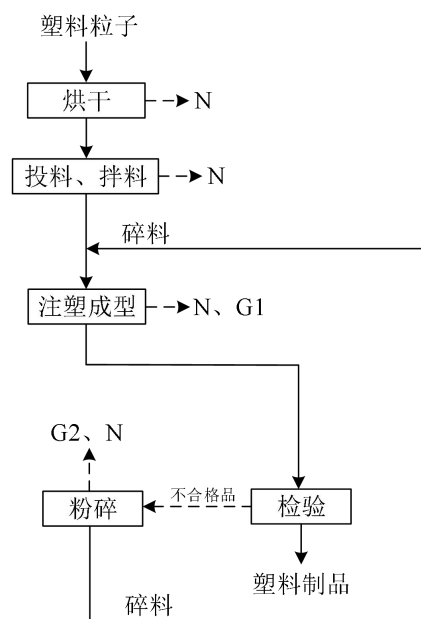
图 2-2 塑料制品生产工艺流程及产污环节图
