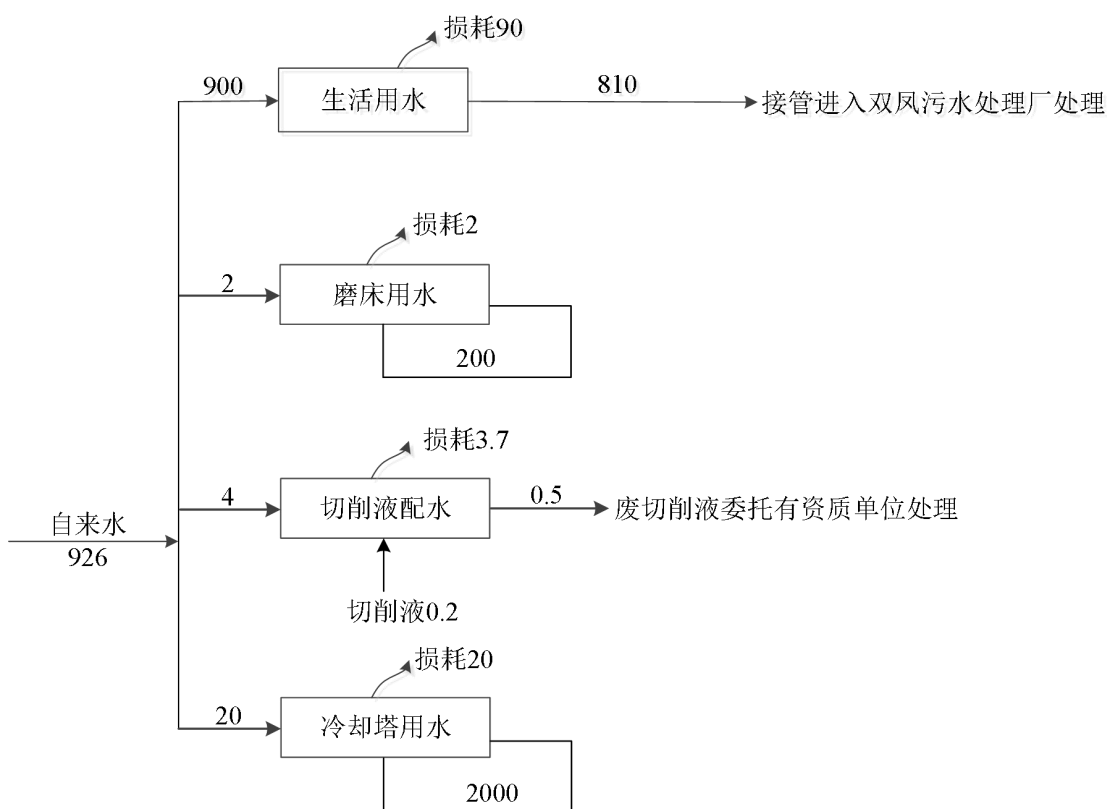
图 2-1 本项目水平衡图 (m³/a)
