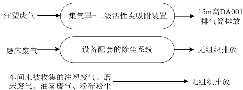
图 4-1 废气处理工艺流程图
