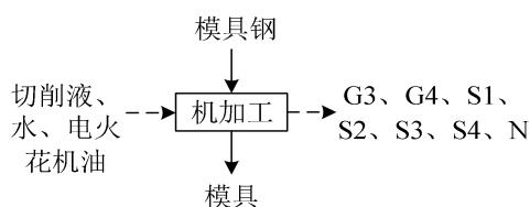
图 2-3 模具生产工艺流程及产污环节图
