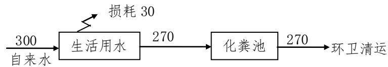
图2 建设项目用排水平衡图 (单位 t/a)
