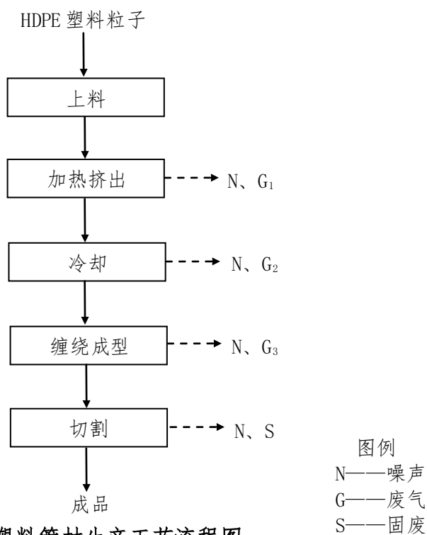
图 1 塑料管材生产工艺流程图
