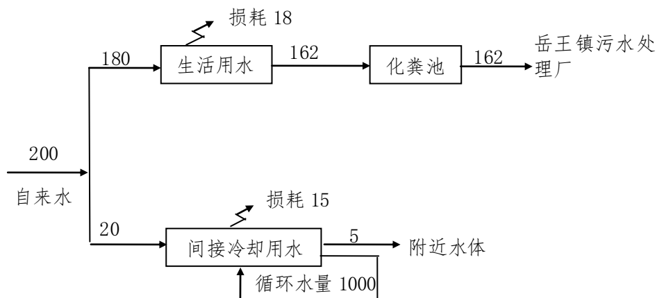
图 4 建设项目用排水平衡图 (单位 t/a)
