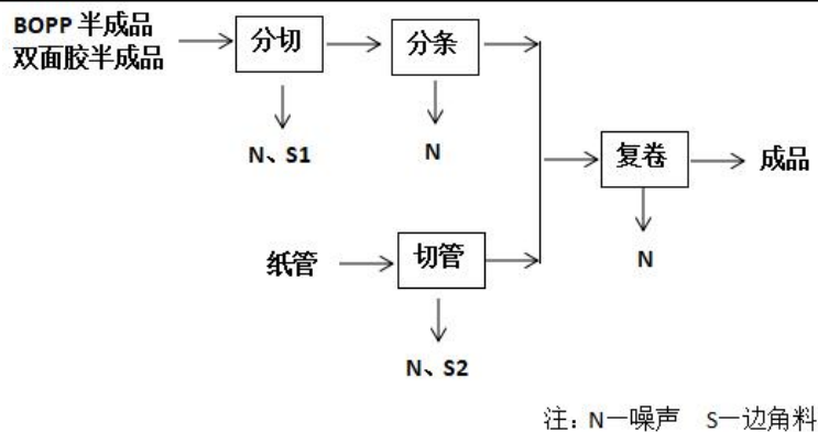
图 2-1 封箱胶带、双面胶带工艺流程及产污环节图
